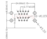
PCB布局 (PCB Layout)
