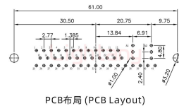
PCB布局 (PCB Layout)
